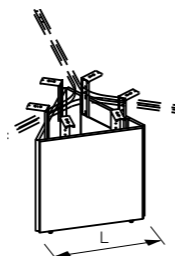
base triangolare per piani 120° 120° top triangular base base triangulaire pour plateaux 120° base con puerta para sobre 120°
